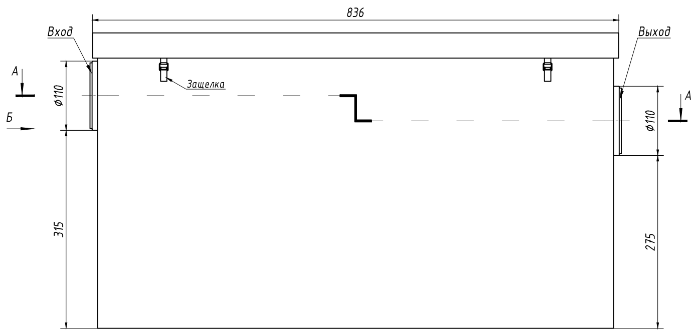
Вид спереди
