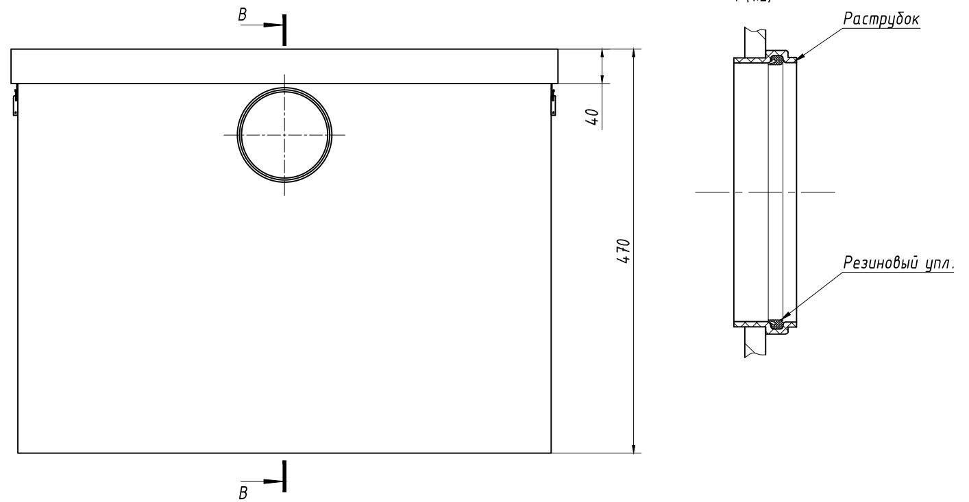
Вид Б
